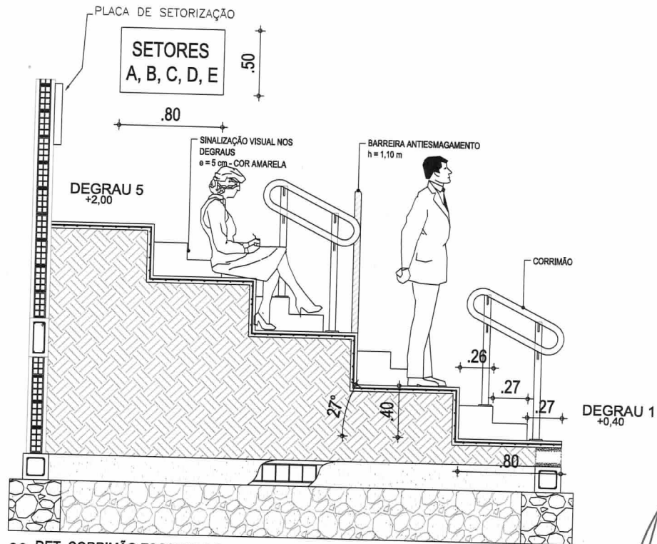
03 DET. CORRIMÃO ESCADAS DE ACESSO ESC.: 1/25
