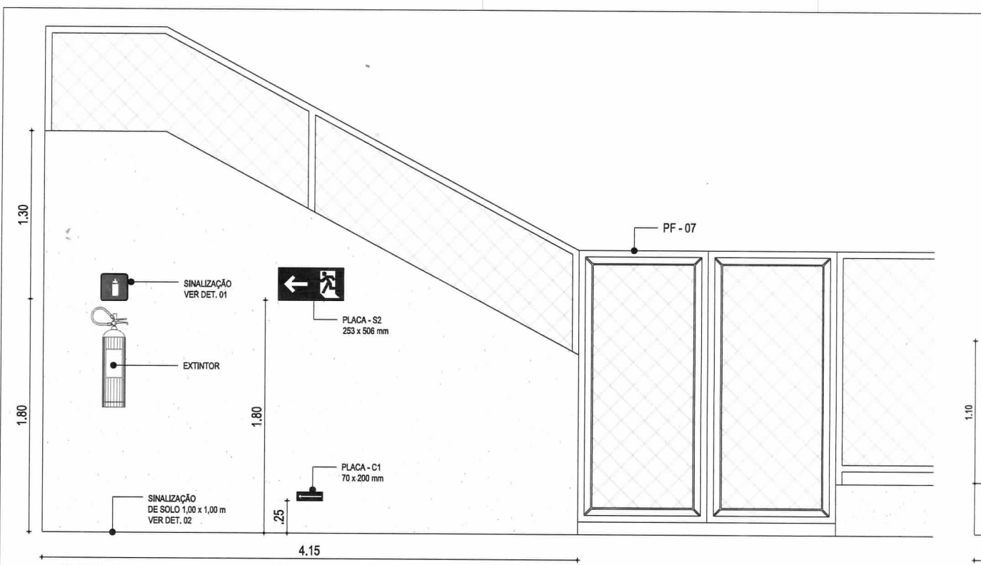
02 DETALHE - EXTINTOR / SINALIZAÇÃO DE EMERGÊNCIA NA ARQUIBANCADA ESC.: 1/25
