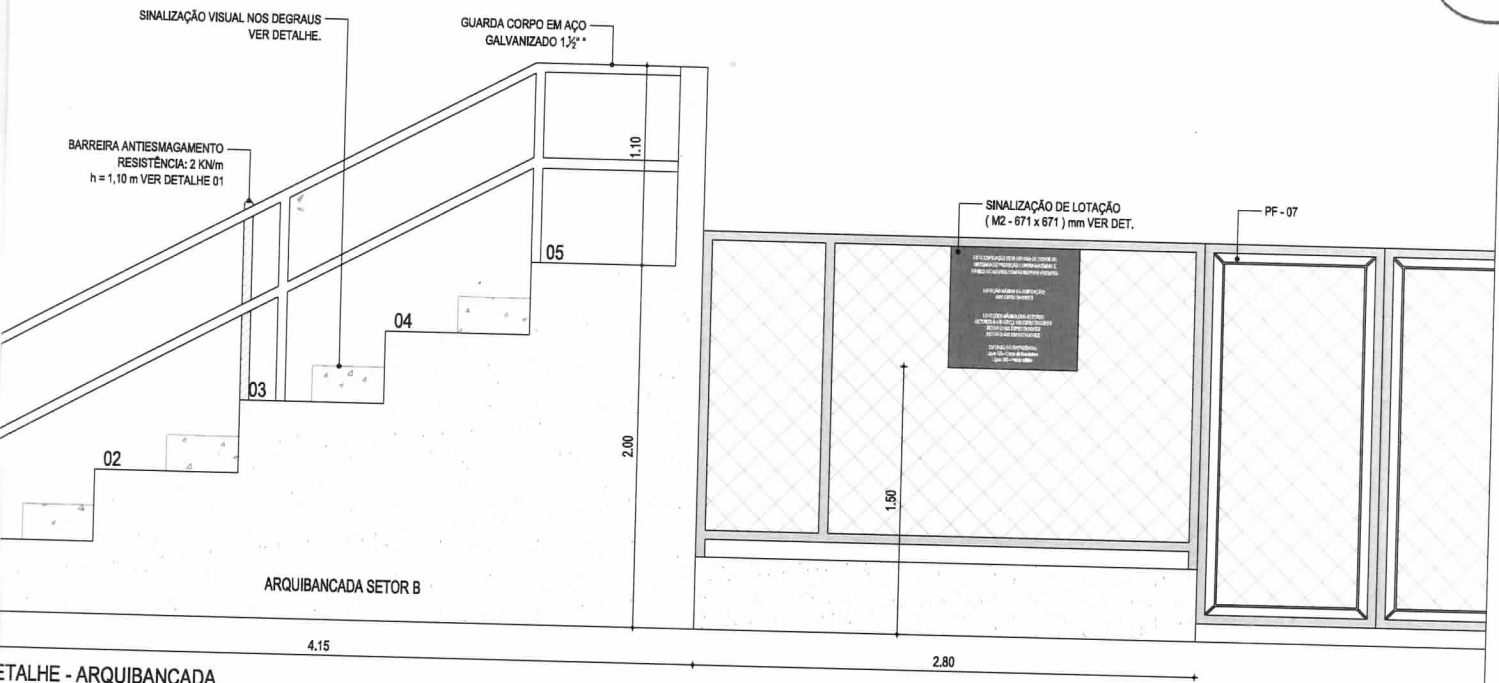
DETALHE - ARQUIBANCADA ESC.: 1/25
