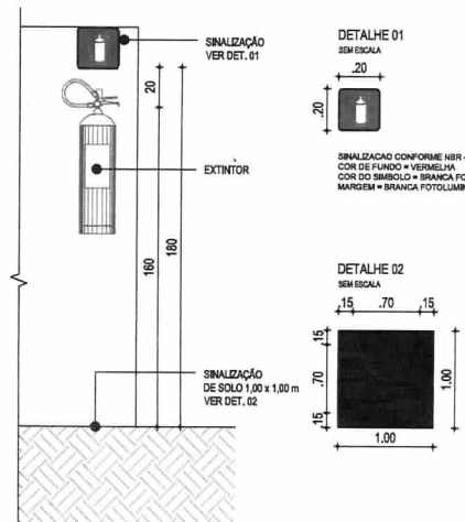
05 DETALHE DOS EXTINTORES ESC.: 1/25
