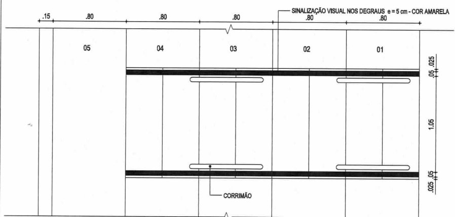
04 DETALHE - SINALIZAÇÃO NAS ESCADAS DE ACESSO ESC.: 1/25
