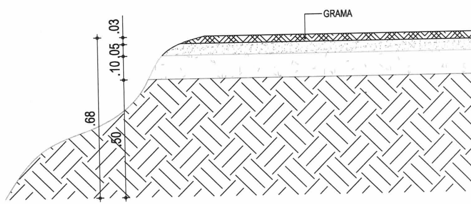
03 CORTE AA - DRENAGEM ESC.: 1/10
