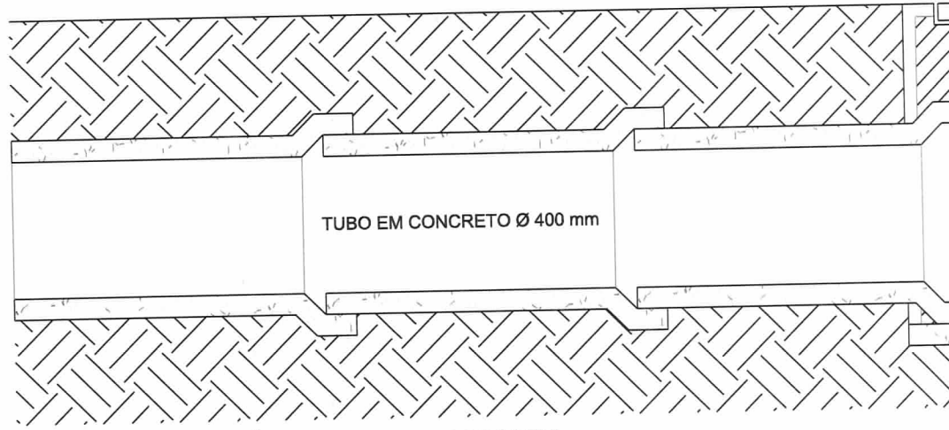
02 DETALHE LIGAÇÃO DA CAIXA DE PASSAGEM ESC.: 1/10
