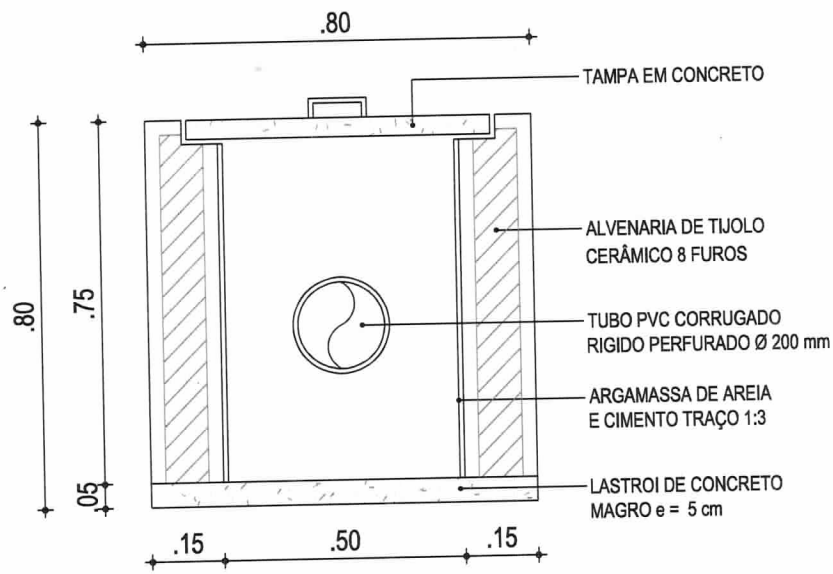
01 DETALHE CAIXA DE PASSAGEM ESC.: 1/10
