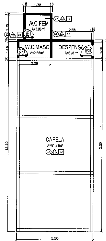
PLANTA BAIXA PROPOSTA esc 1:100
