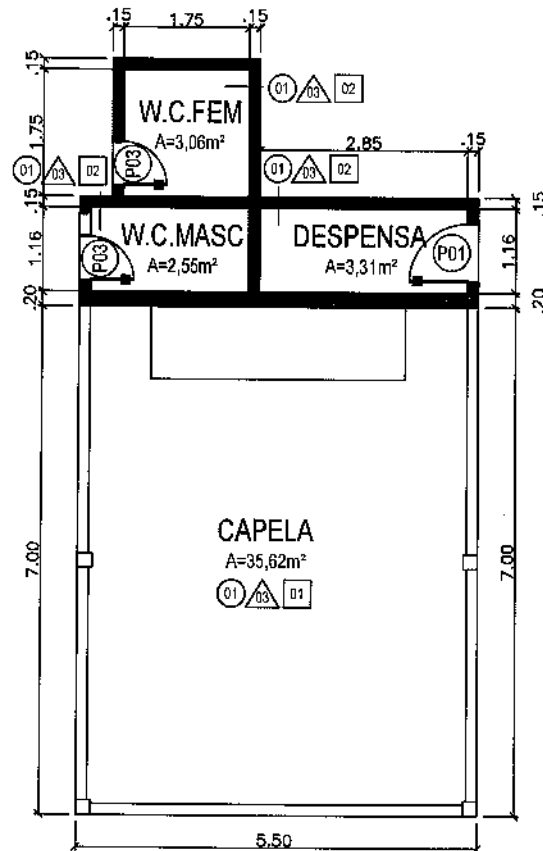
PLANTA BAIXA EXISTENTE esc 1:100
