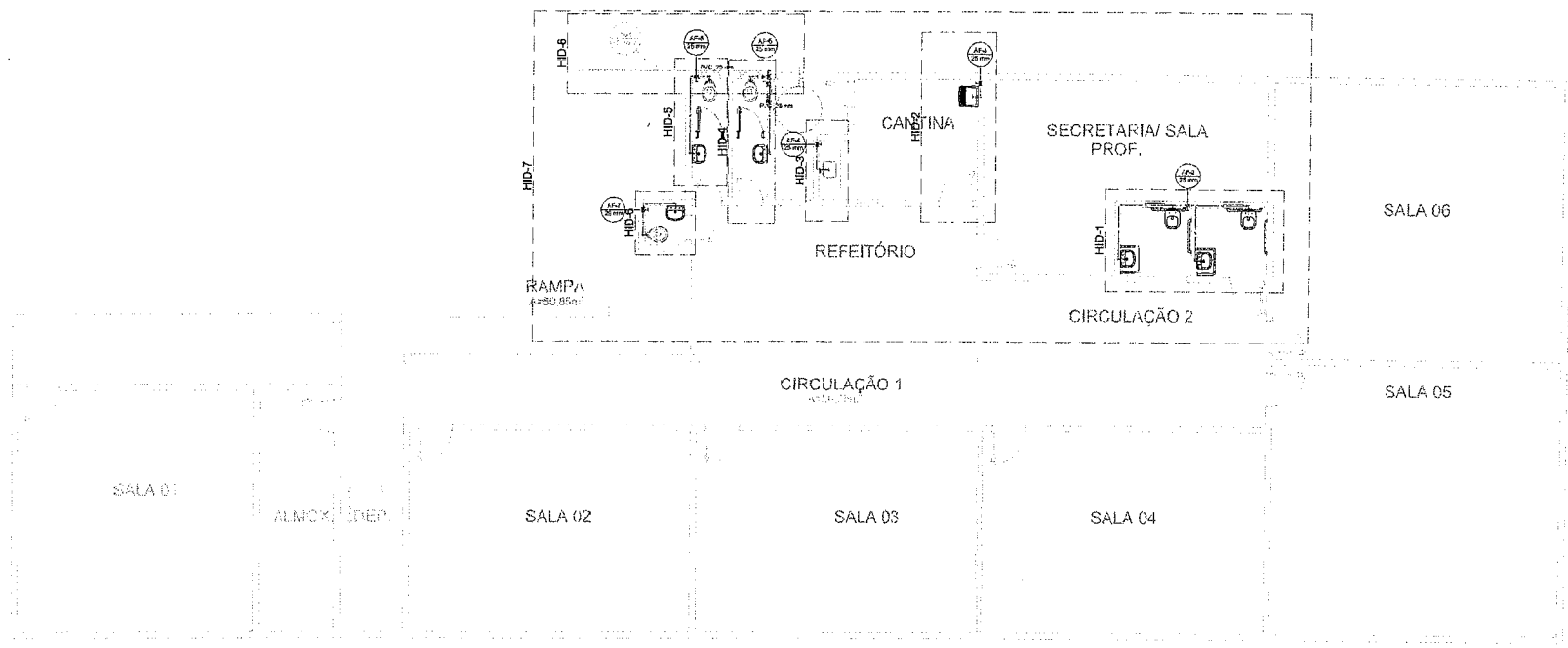
01 PLANTA BAIXA - HIDRÁULICO ESC: 1/25
