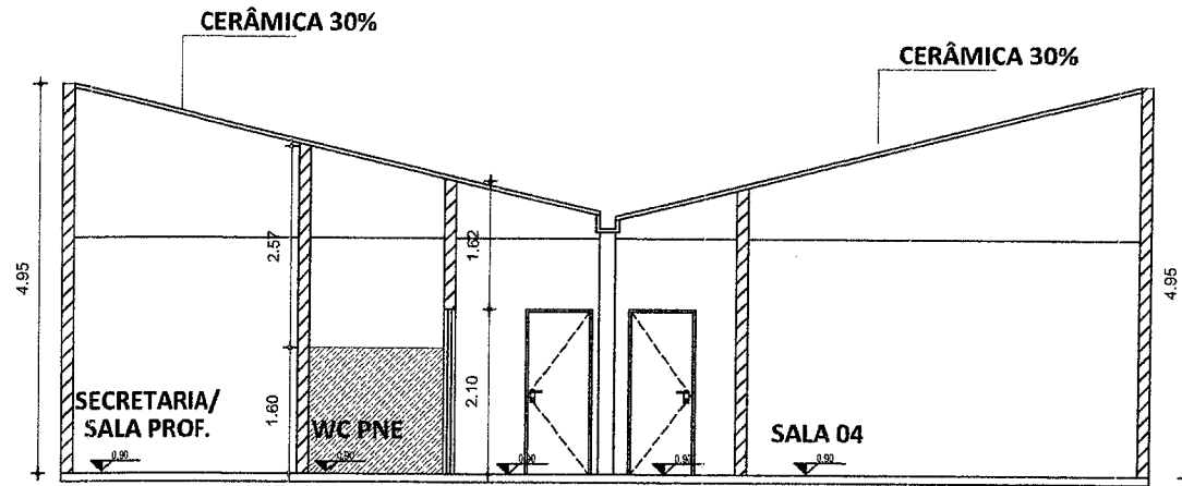
06 | PLANTA CORTE: B-B ESC.: 1/75
