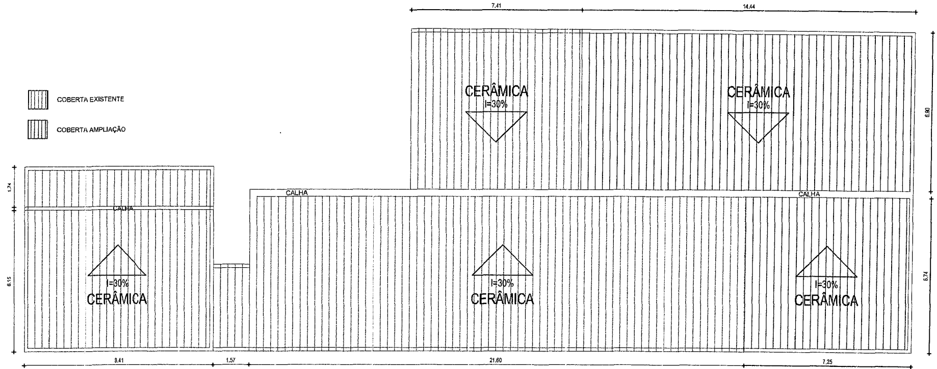
04 | PLANTA DE COBERTA ESC.: 1/120
