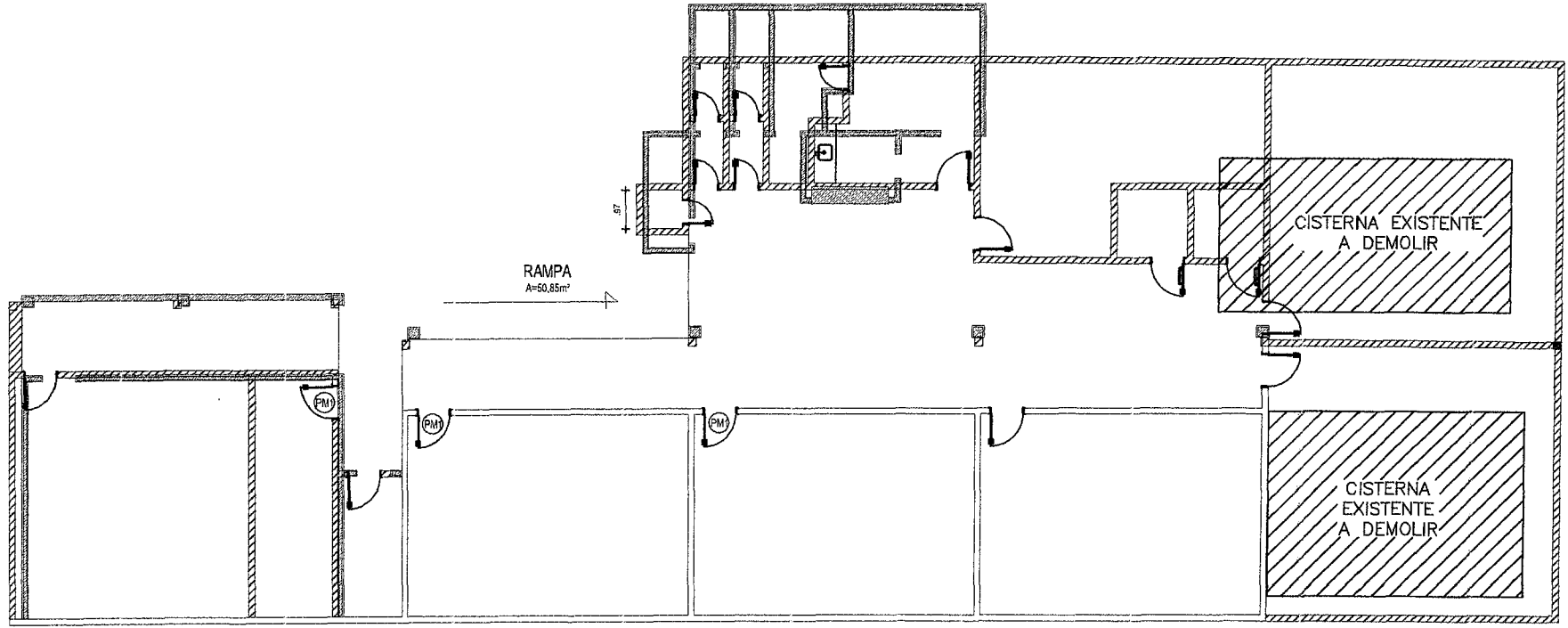
05 PLANTA BAIXA - CONSTRUIR E DEMOLIR ESC: 1/100
